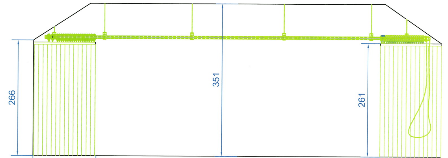
Kurtyna główna - detale
