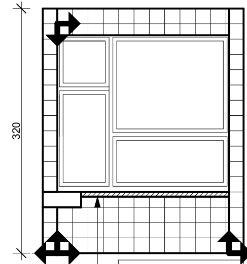
RŚ-03/03
