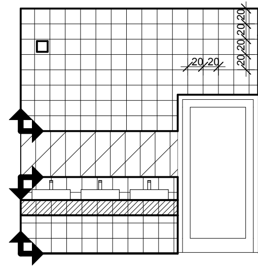
RŚ-04/02 1:50
