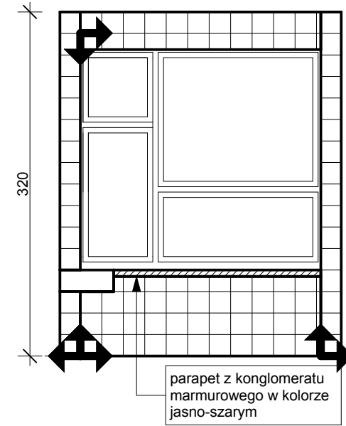
RŚ-03/03 1:50
