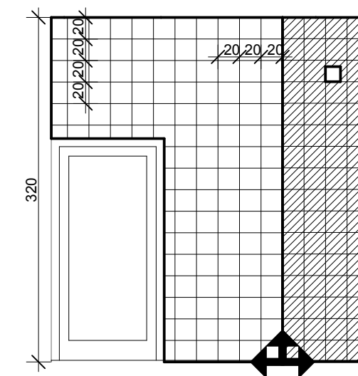
RŚ-05/04 1:50
