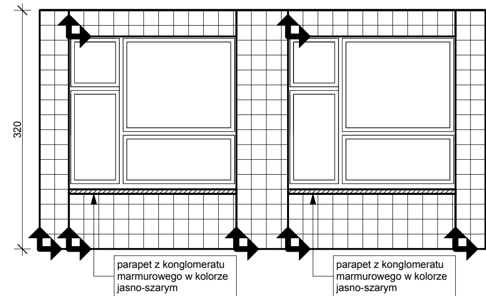
RŚ-05/04 1:50
