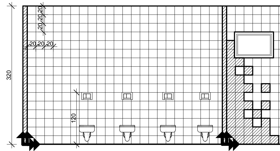
RŚ-05/01 1:50
