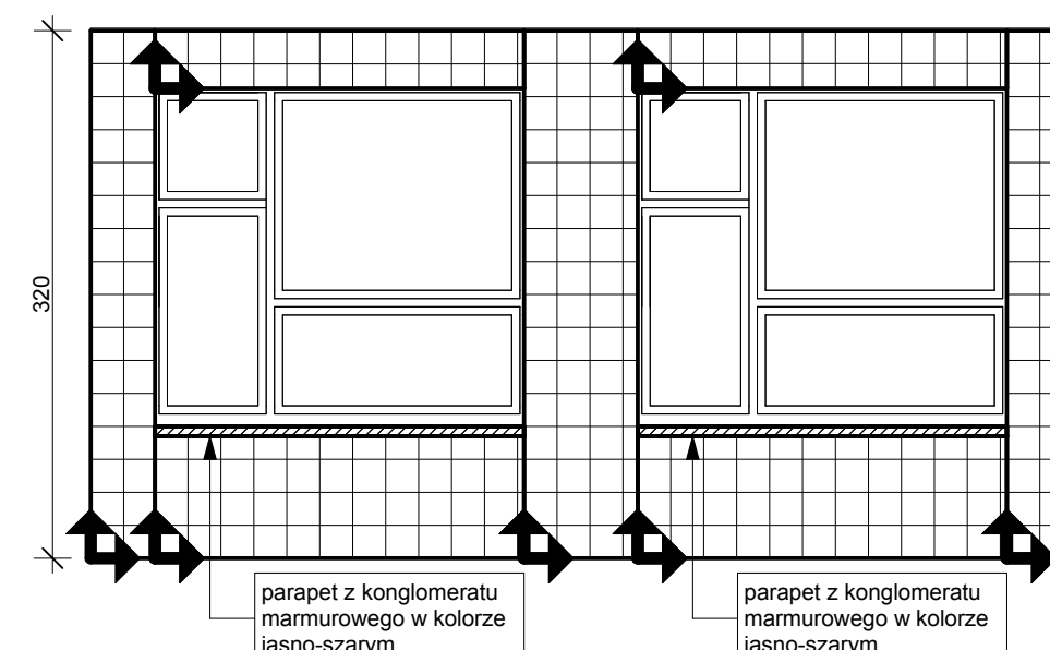
RŚ-05/03 1:50
