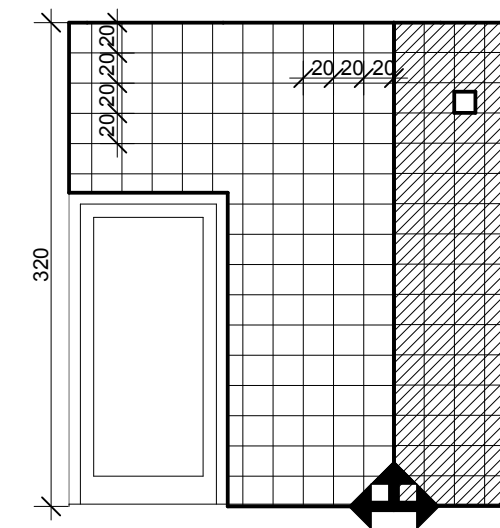
RŚ-05/04 1:50
