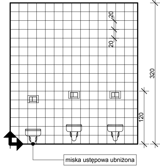
RŚ-02/01 1:50
