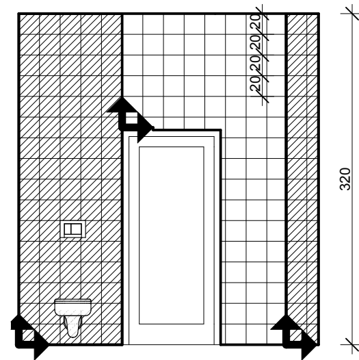
RŚ-01/01
