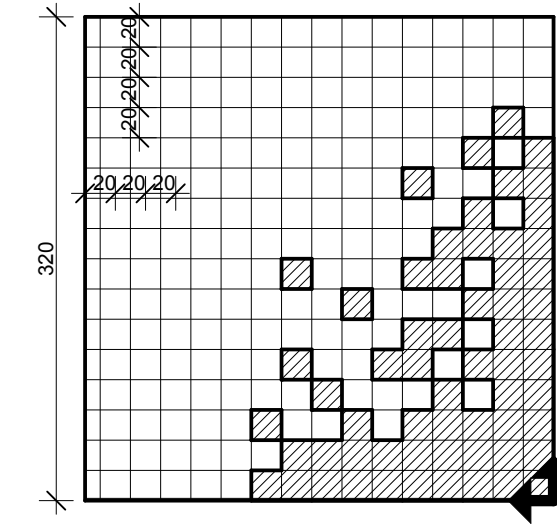
RŚ-04/04 1:50
