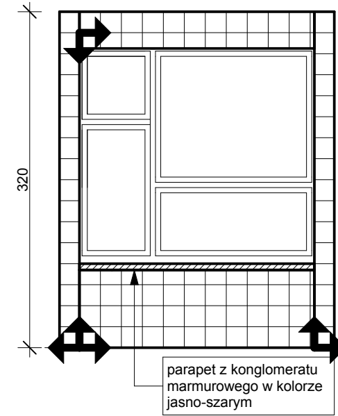
RŚ-05/02 1:50
