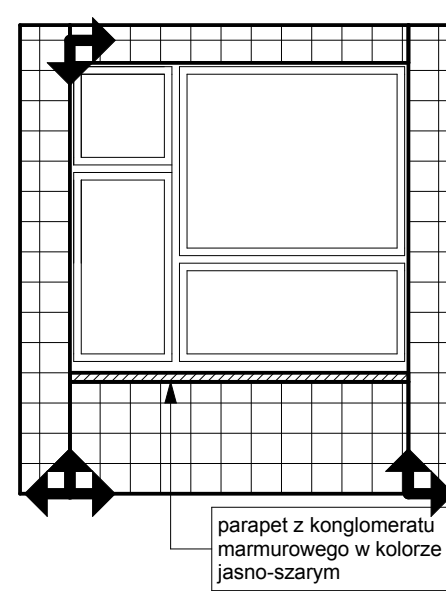
RŚ-02/03 1:50
