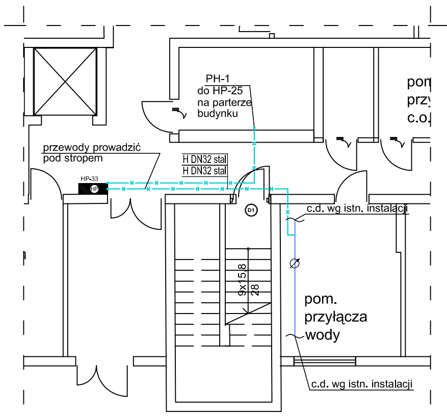
RZUT PRZYZIEMIA
